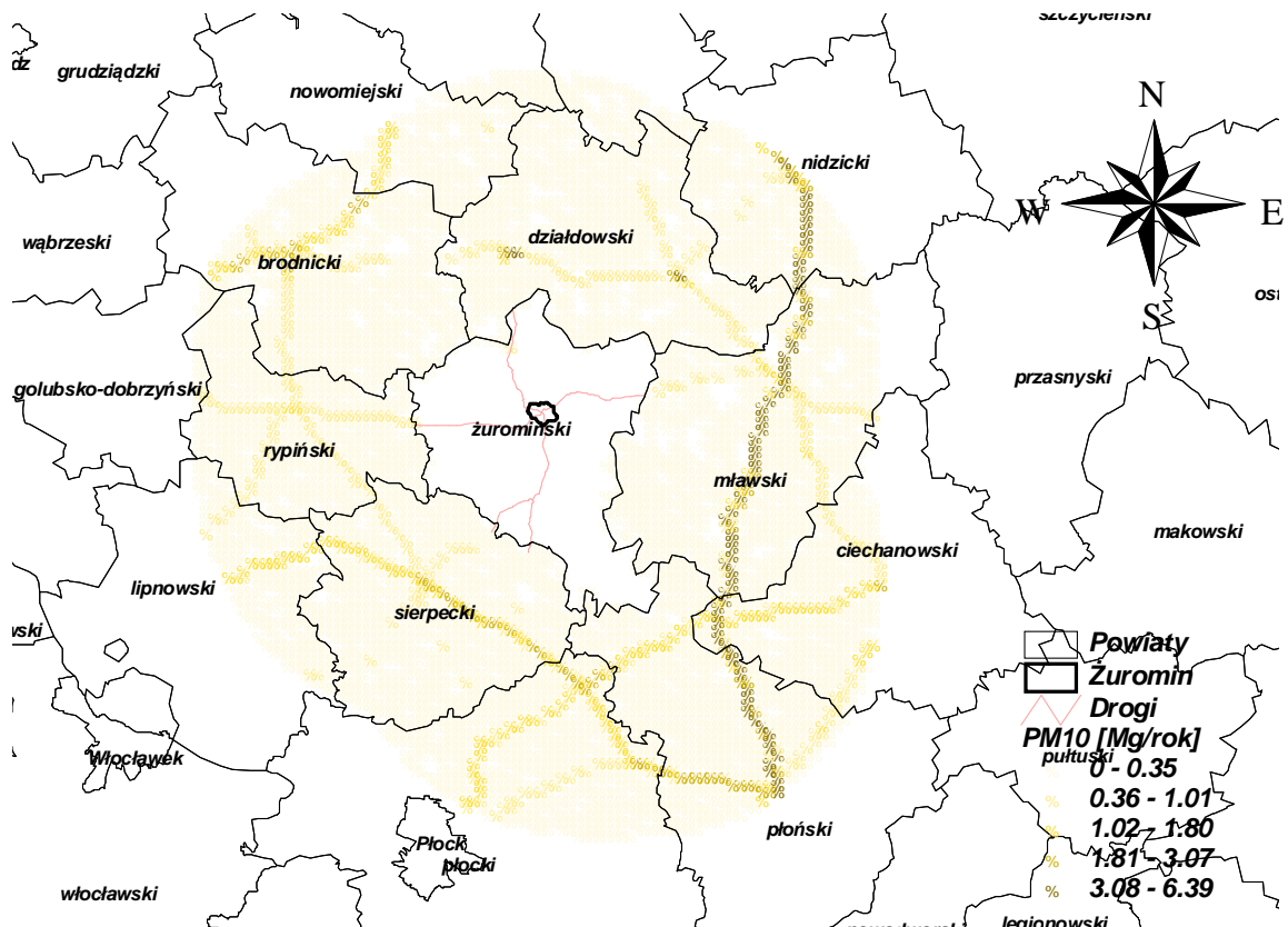
Rysunek 3.5 Całkowita emisja pyłu zawieszonego PM10 ze źródeł liniowych zlokalizowanych w pasie 30 km od powiatu żuromińskiego w 2005 roku.
