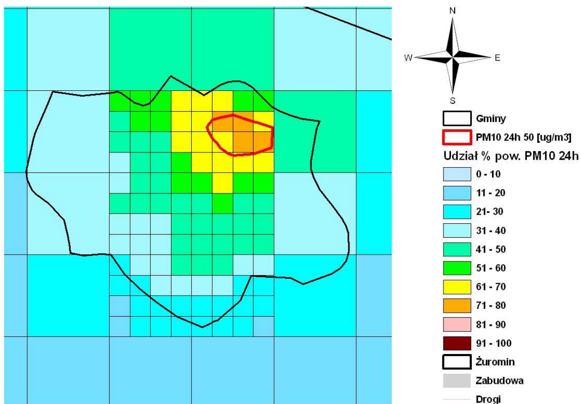
Rysunek 4.3 Udział procentowy emisji powierzchniowej w stężeniach całkowitych pyłu zawieszono PM10 o okresie uśredniania wyników pomiarów 24 godziny w Żurominie w 2005 roku.
