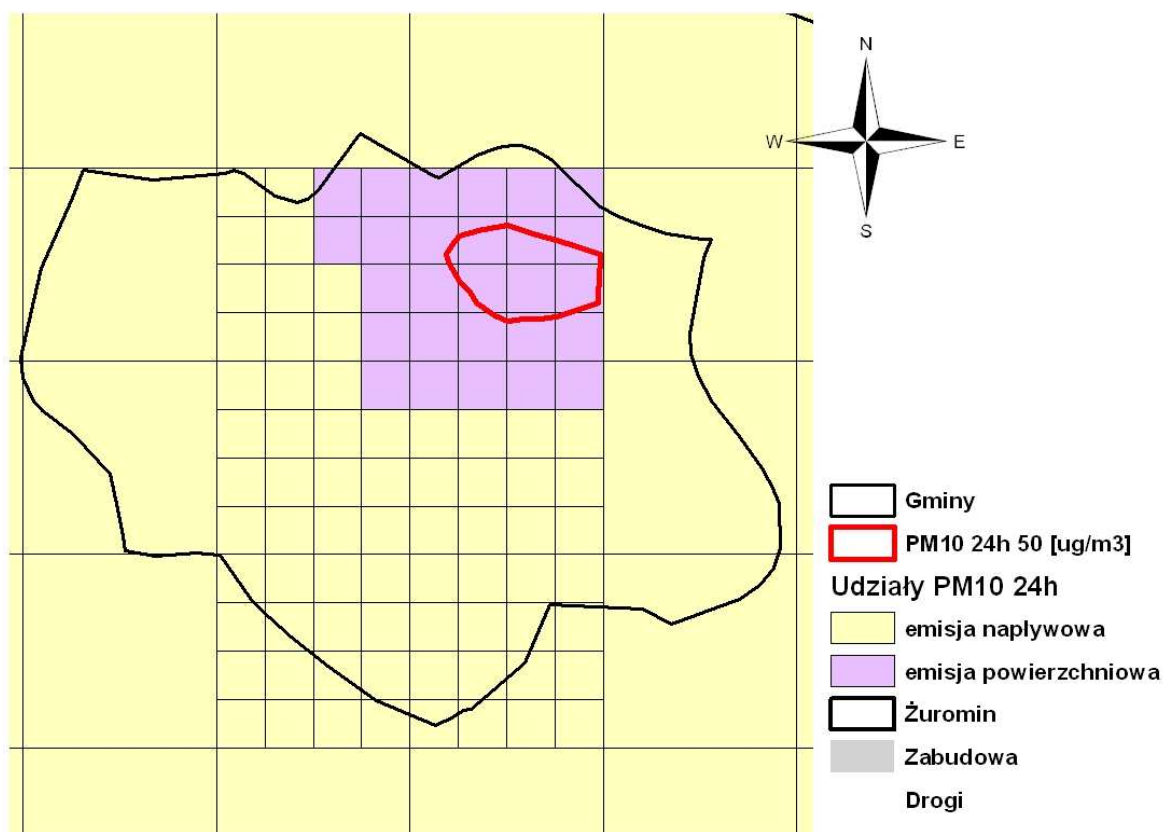
Rysunek 4.2 Większościowy udział poszczególnych typów emisji w stężeniach pyłu zawieszono PM10 o okresie uśredniania wyników pomiarów 24 godziny w Żurominie w 2005 roku – obszar przekroczeń pyłu zawieszono PM10 o okresie uśredniania wyników pomiarów 24 godziny od emisji całkowitej.
