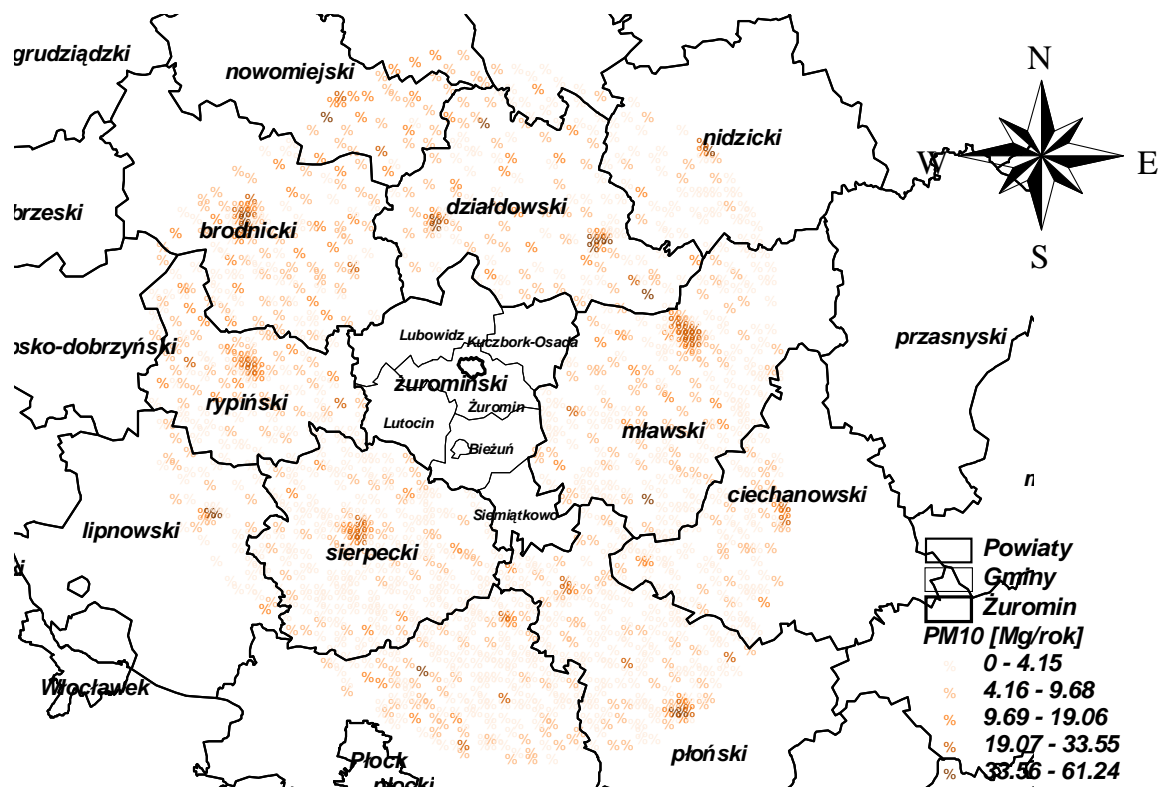
Rysunek 3.4 Emisja pyłu zawieszono PM10 ze źródeł powierzchniowych zlokalizowanych w pasie 30 km od powiatu żuromińskiego w 2005 roku.
