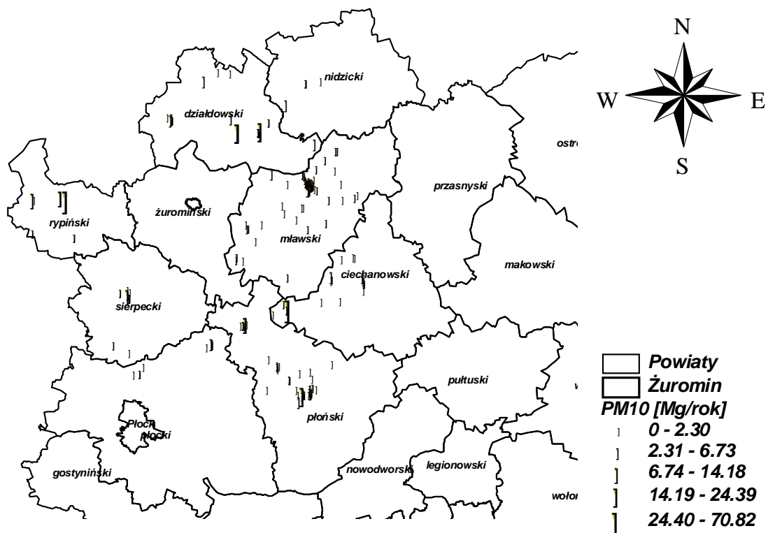
Rysunek 3.3 Emisja pyłu zawieszono PM10 z emitorów punktowych zlokalizowanych w pasie 30 km od powiatu żuromińskiego 2005 roku.
