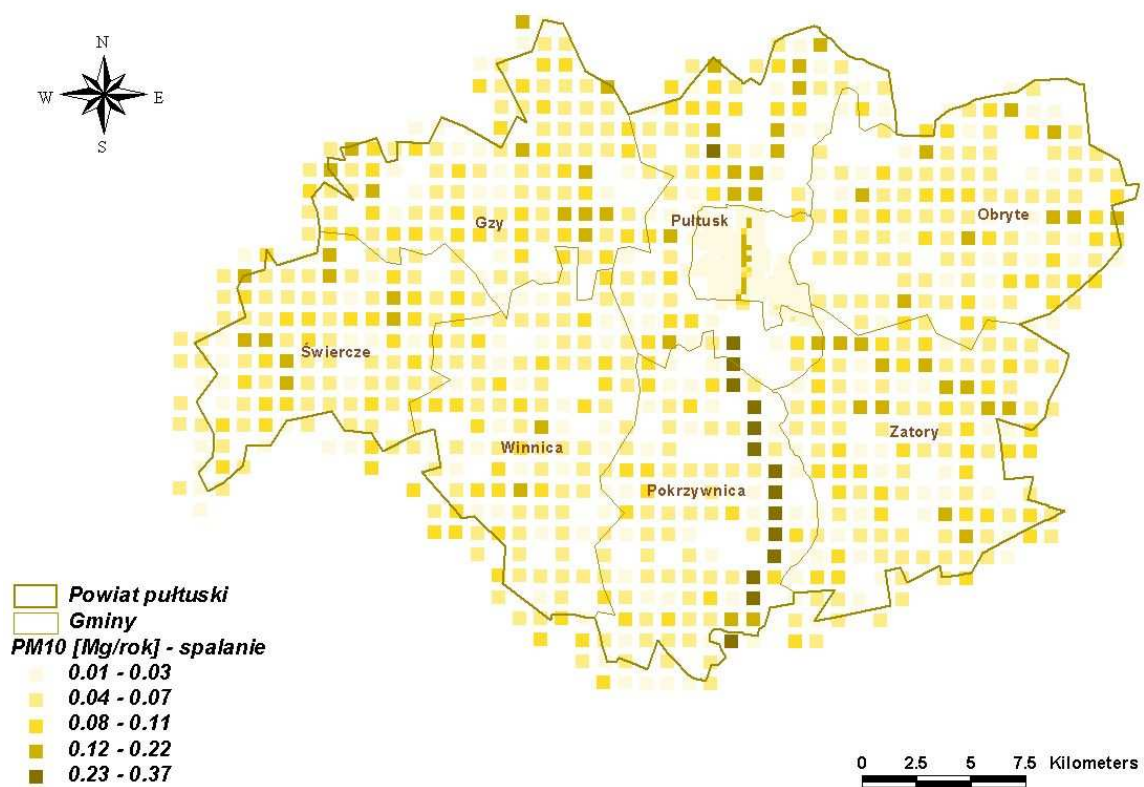
Rysunek 3.16 Emisja pyłu zawieszonego PM10 ze spalania paliw, ze źródeł komunikacyjnych w powiecie pultuskim w 2006 roku
