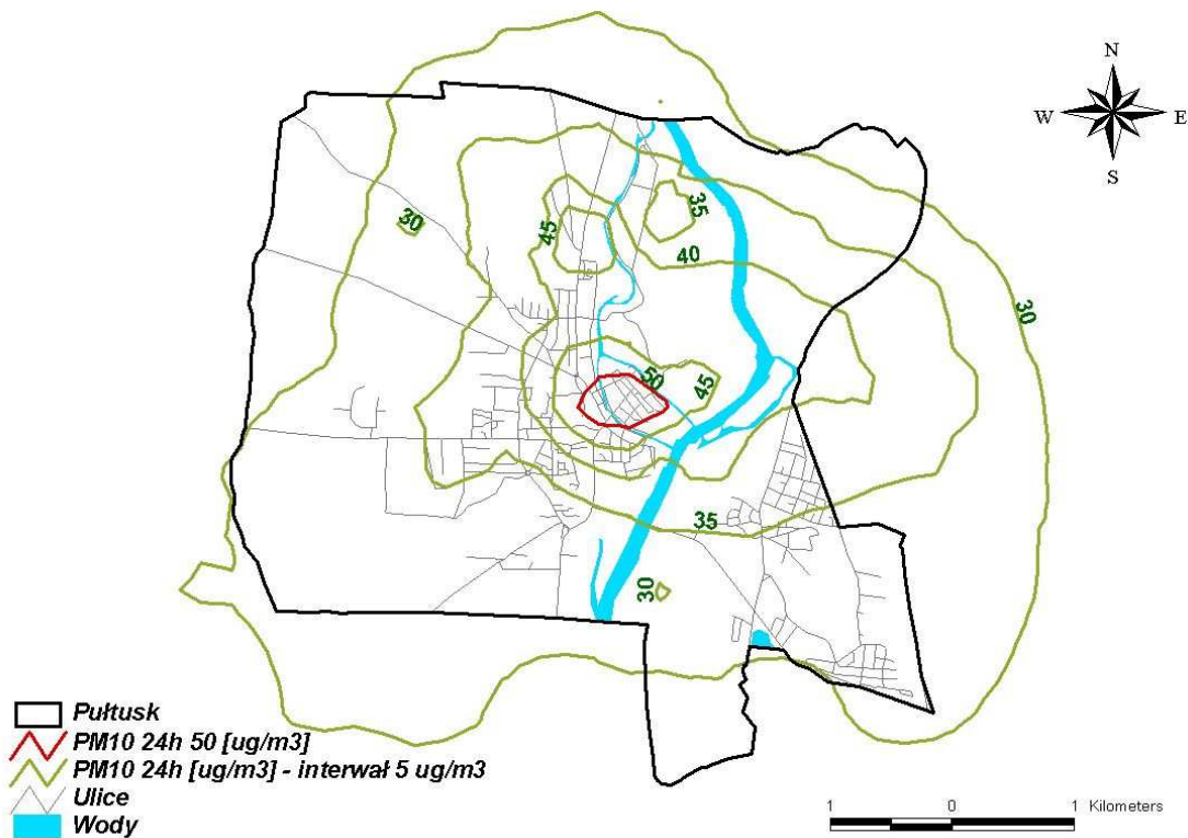
Rysunek 7.1 Rozkład stężeń pyłu zawieszonego PM10 o okresie uśredniania wyników pomiarów 24 godziny, powodowanych emisją całkowitą, po zrealizowaniu I etapu
