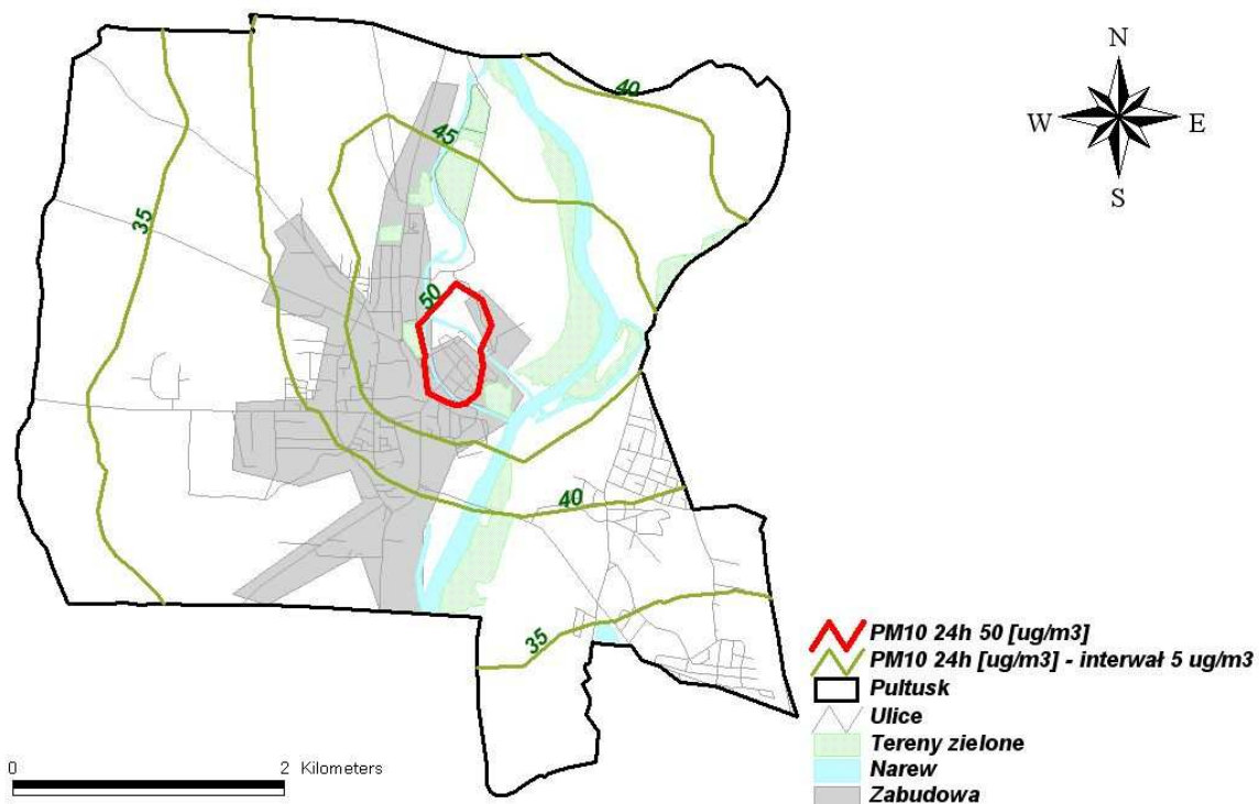
Rysunek 6.1 Zasięg obszaru miasta Pułtusk, na którym należy prowadzić działania naprawcze
