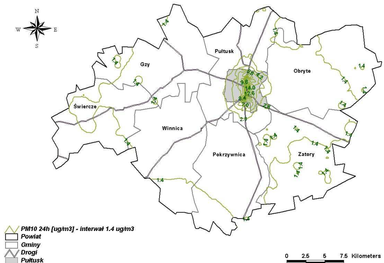
Rysunek 3.49 Rozkład stężeń pyłu zawieszonego PM10 o okresie uśredniania wyników pomiarów 24 godziny pochodzących od emisji komunikacyjnej, w powiecie pułtuskim w 2006 roku
