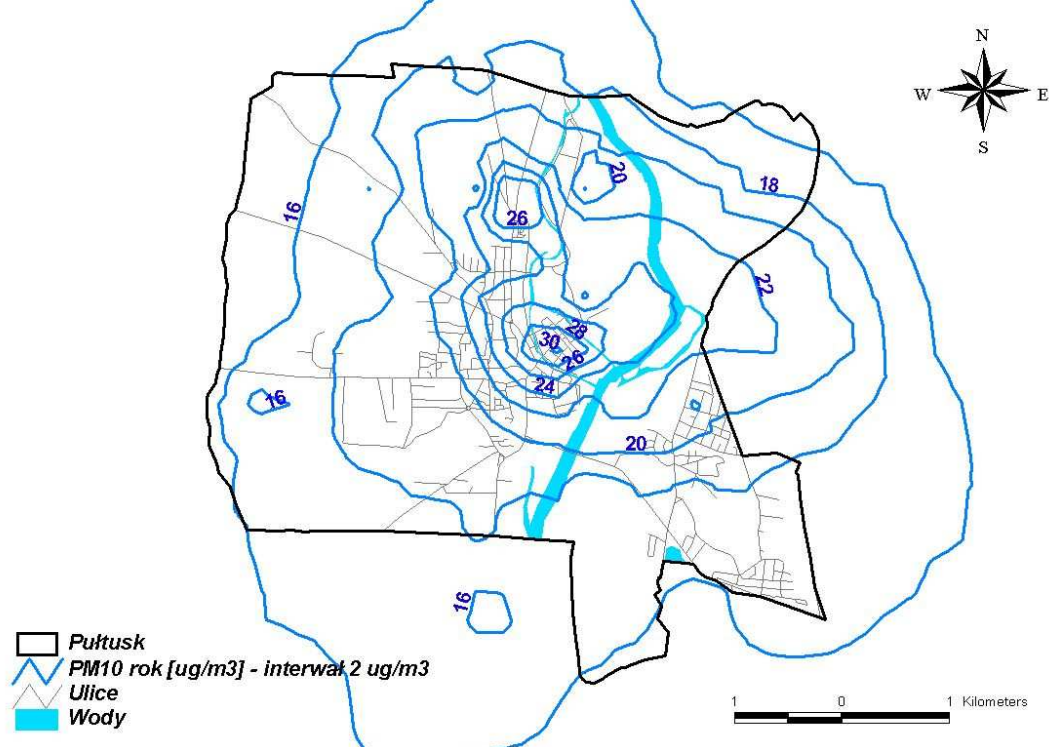
Rysunek 7.2 Rozkład stężeń pyłu zawieszonego PM10 o okresie uśredniania wyników pomiarów rok kalendarzowy, powodowanych emisją całkowitą, po zrealizowaniu I etapu
