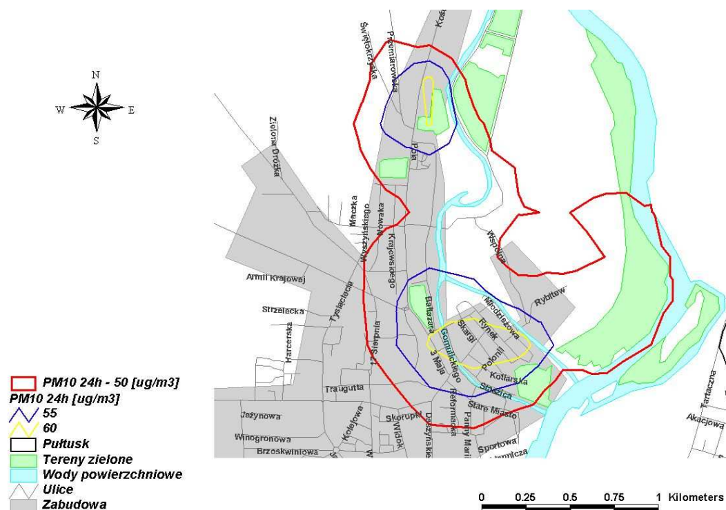
Rysunek 4.1 Obszar przekroczeń poziomu dopuszczalnego stężeń pyłu zawieszono PM10 o okresie uśredniania wyników pomiarów 24 godziny, w obrębie izolinii 50 µg/m 3 , w Pułtusku, w 2006 roku
