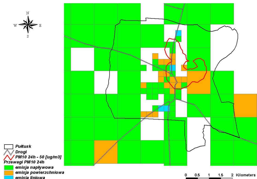
Rysunek 4.2 Przewagi poszczególnych typów emisji w stężeniach całkowitych pyłu zawieszono PM10 o okresie uśredniania wyników pomiarów 24 godziny, w powiecie pułtuskim w 2006 roku
