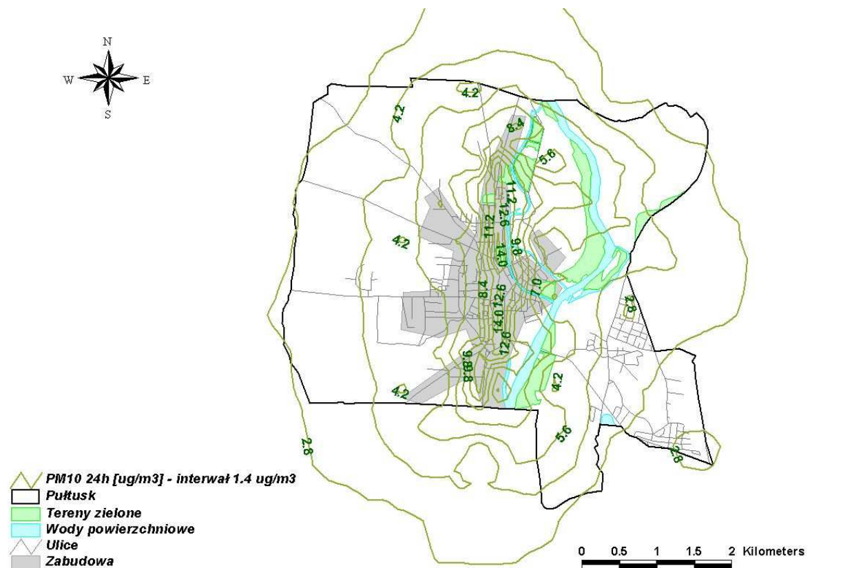
Rysunek 3.50 Rozkład stężeń pyłu zawieszonego PM10 o okresie uśredniania wyników pomiarów 24 godziny pochodzących od emisji komunikacyjnej, w Pułtusku w 2006 roku
