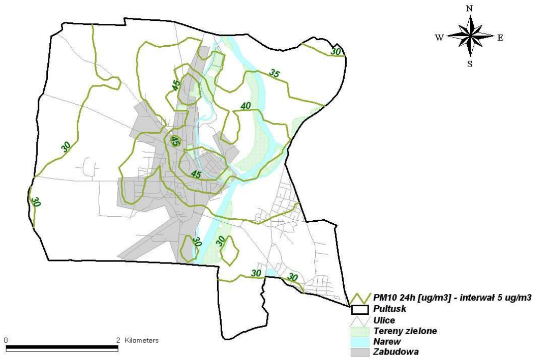
Rysunek 7.3 Rozkład stężeń pyłu zawieszonego PM10 o okresie uśredniania wyników pomiarów 24 godziny, pochodzących od całkowitej emisji, po zastosowaniu działań naprawczych
