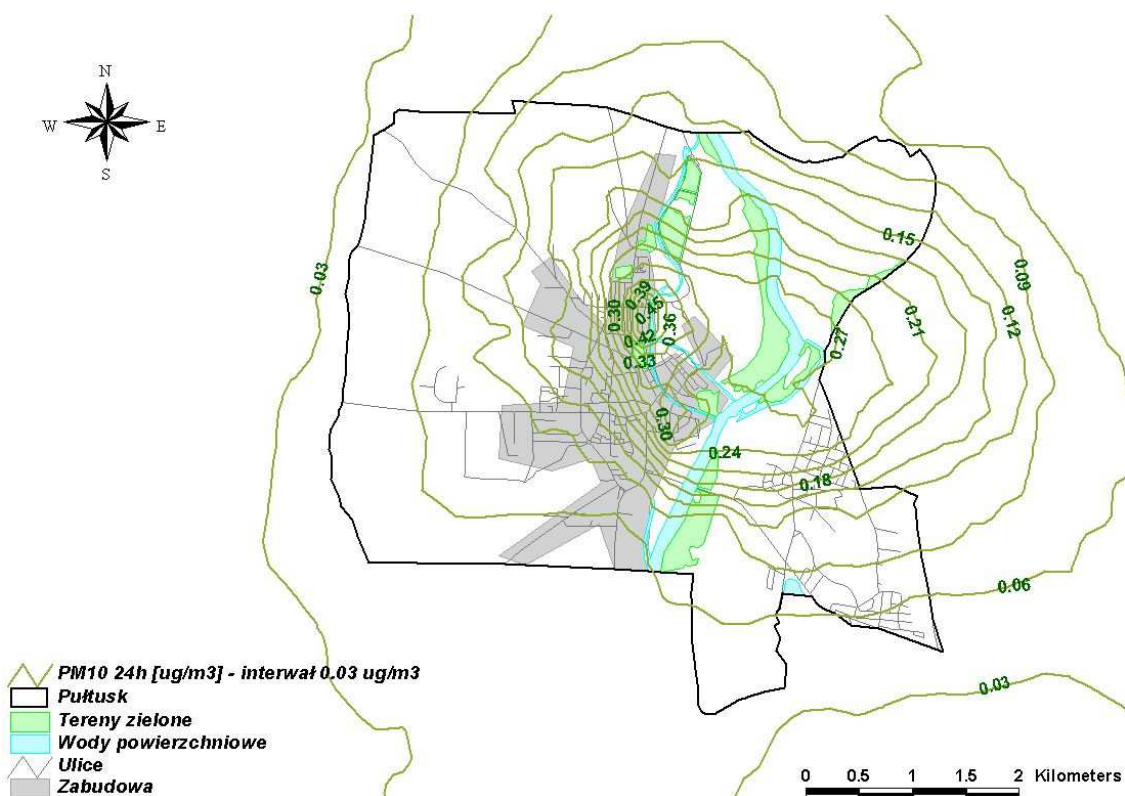
Rysunek 3.42 Rozkład stężeń pyłu zawieszonego PM10 o okresie uśredniania wyników pomiarów 24 godziny pochodzących od emisji punktowej, w Pułtusku, w 2006 roku
