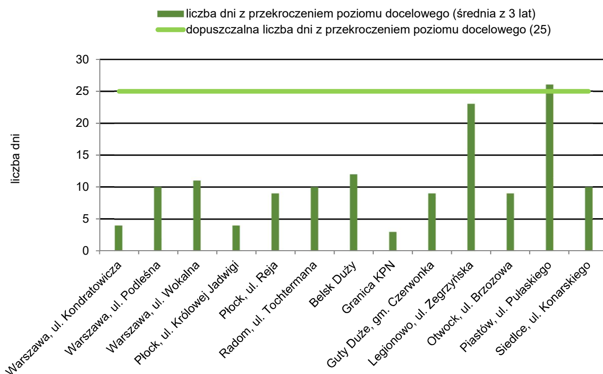
Rysunek 8 Wartości stężeń ozonu w województwie mazowieckim w latach 2014–2016 roku [źródło: WIOŚ]
