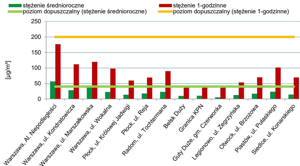
Rysunek 2 Wartości stężeń \text{NO}_2 w województwie mazowieckim w 2016 roku [źródło: WIOŚ]
